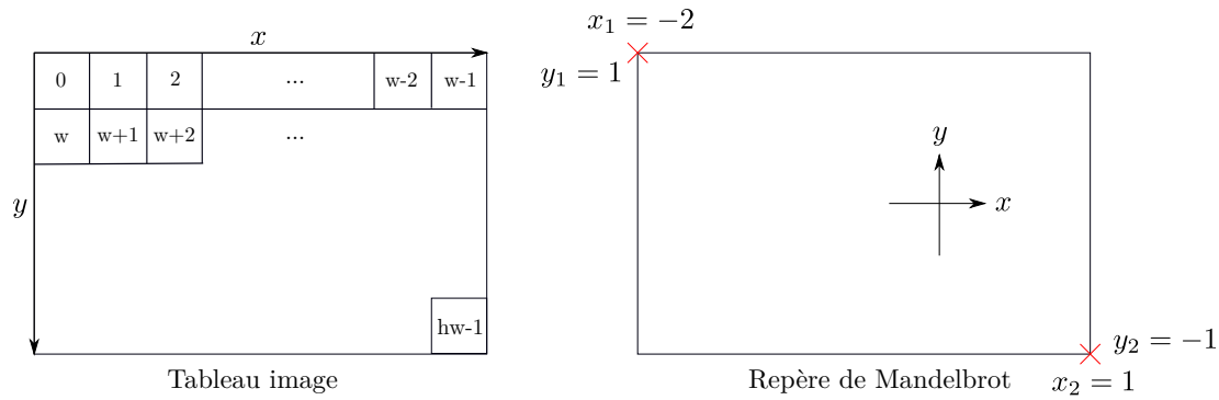
Figure 2: Visualisation du repère de Mandelbrot dans le cas x_1 = -2 , y_1 = 1 , et x_2 = 1 , y_2 = -1 .
