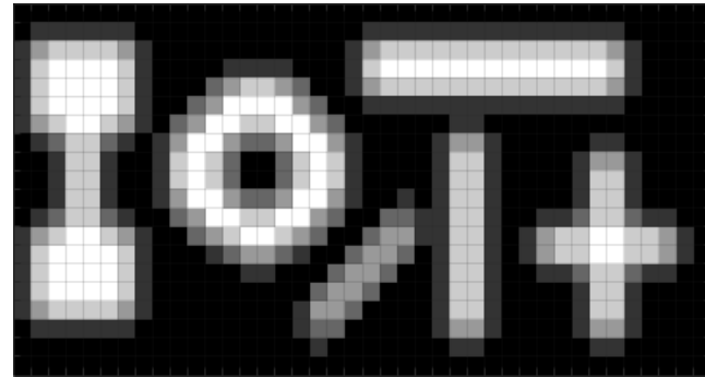
Image convoluée I_c
